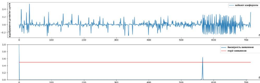
Рисунок 1 - Аналіз часових рядів аномального трафіку
