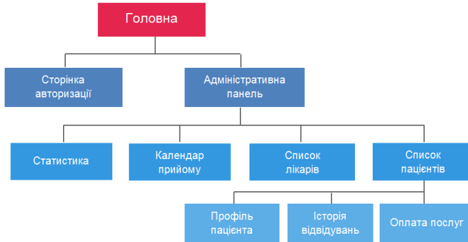
Рисунок 1 – Структура сторінок
