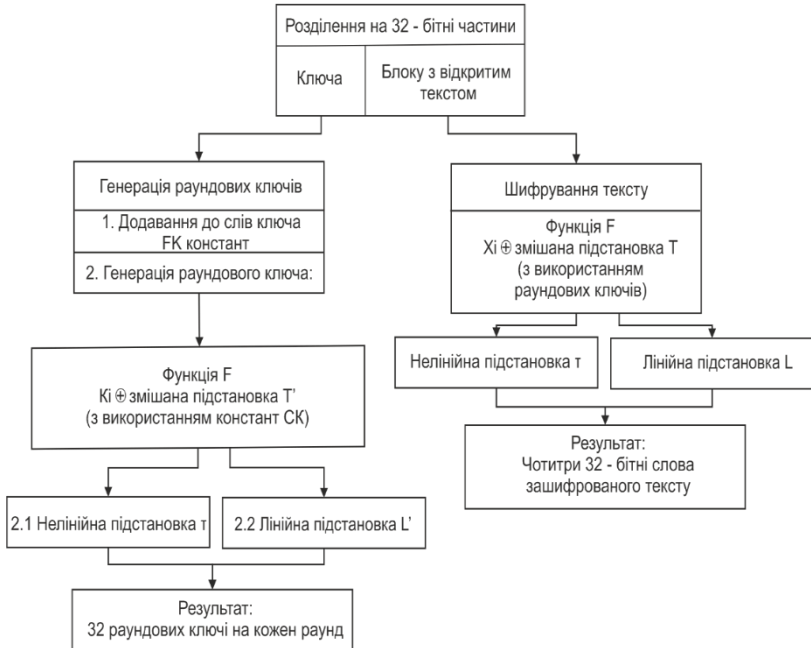
Рисунок 1 – Алгоритм шифрування стандарту SM4
