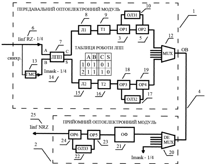
Риунок 1 Пристрій маскування конфіденційної інформації
